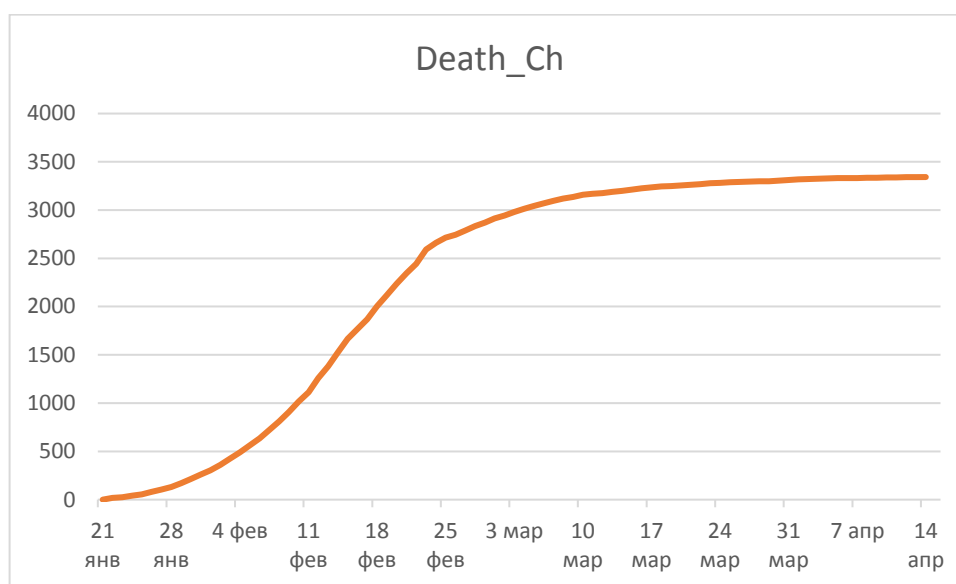
Рисунок 5 – Данные о количестве умерших от коронавируса в Китае
