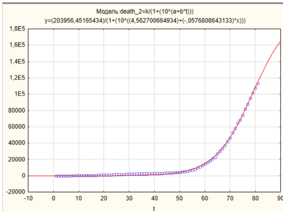
Рисунок 1 – График по полученной спецификации (красный) и реальные данные (синие) для параметра Death по всему миру
