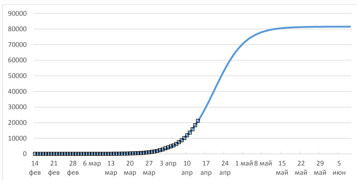
Рисунок 11 – Прогноз по заболеваемости в России по формуле (11)
